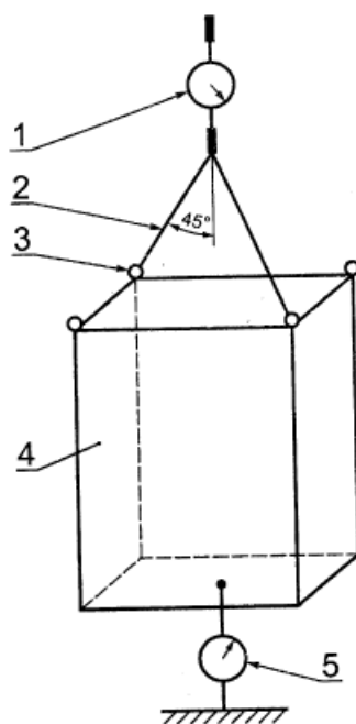
1 — динамометр 1; 2 — строп; 3 — строповое устройство; 4 — ВРУ; 5 — динамометр 2
